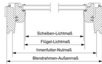
Längsschnitt
