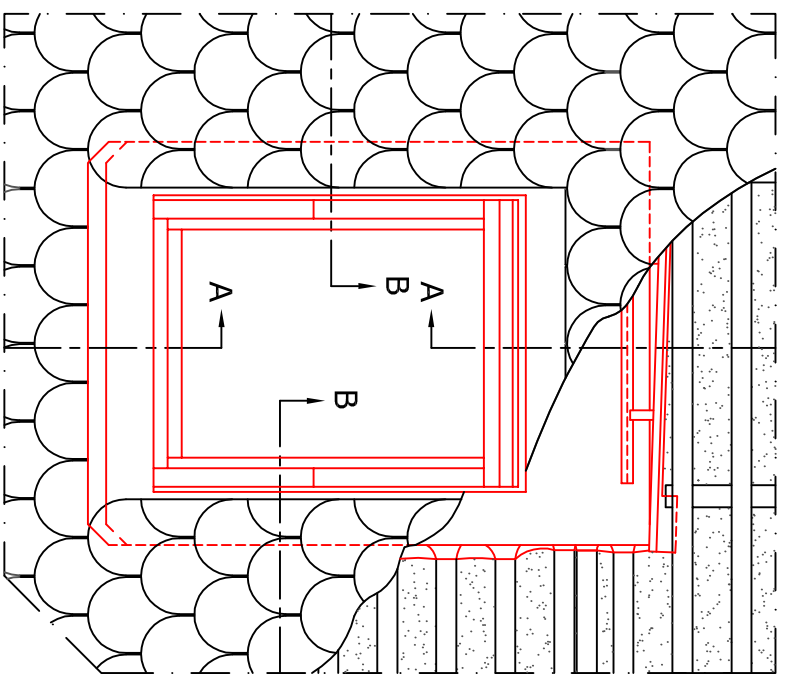
Elevation perpendiculaire au toit
