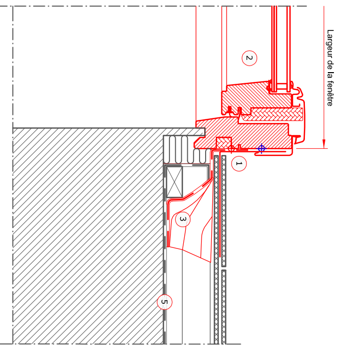
Coupe B-B 1:5
