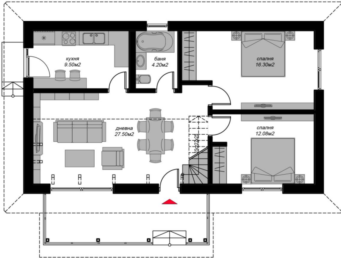
Разпределение кота ±0.00
