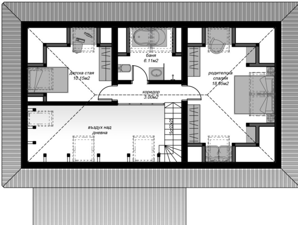
Разпределение кота +3.25
