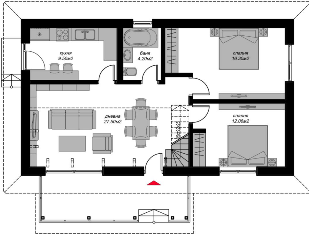
Разпределение кота ±0.00
