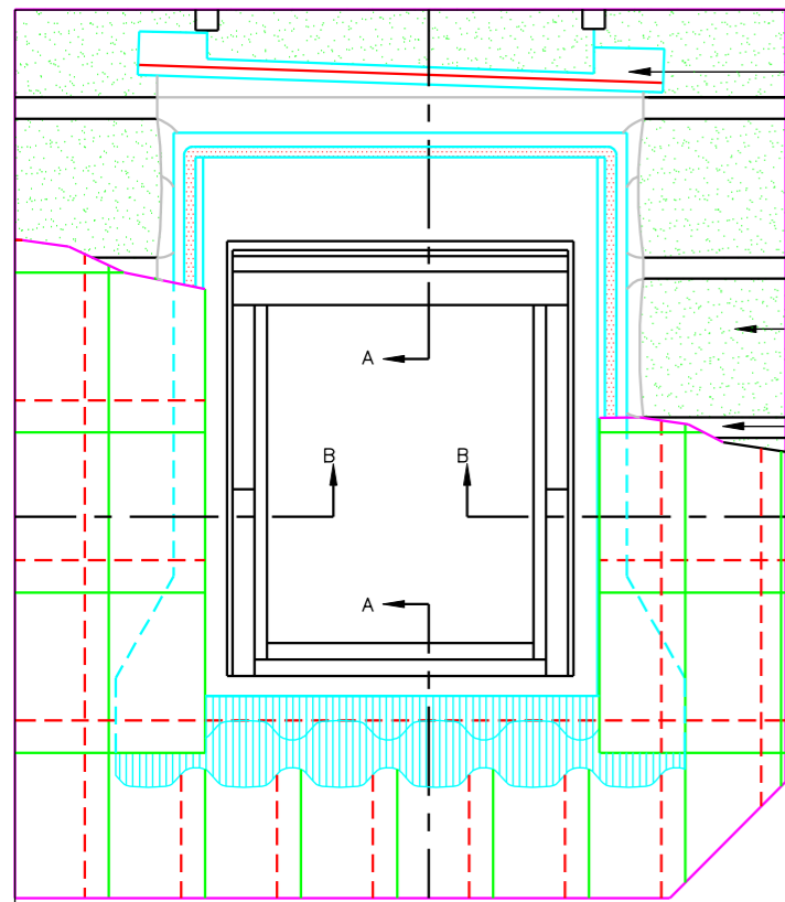
Plan en élévation à angle droit 1:20
