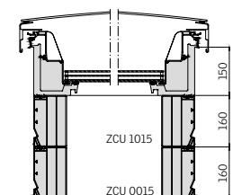
Flachdach-Fenster CVU/CFU mit Aufsetzkranz ZCU 0015 und ZCU 1015
