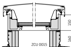
Flachdach-Fenster CVU/CFU mit Aufsetzkranz ZCU 0015
