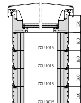
Flachdach-Fenster CVU/CFU mit Aufsetzkranz-Set ZCU S000, bestehend aus Aufsetzkranz ZCU 0015 und ZCU 1015 + zusätzliche Aufsetzkranz-Adapter ZCU 1015. Es können bis zu drei Aufsetzkranz-Adapter ZCU 1015 gestapelt werden.
