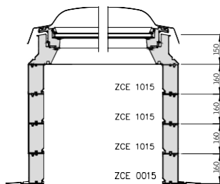
Flachdach-Fenster CVP/CFP mit Aufsetzkranz-Set ZCE S000, bestehend aus Aufsetzkranz ZCE 0015 und ZCE 1015 + zusätzliche Aufsetzkranz-Adapter ZCE 1015. Es können bis zu drei Aufsetzkranz-Adapter ZCE 1015 gestapelt werden. Maximale Höhe 790 mm.
