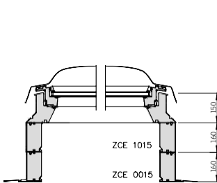
Flachdach-Fenster CVP/CFP mit Aufsetzkranz ZCE 0015 und ZCE 1015 Set-Ausführung ZCE S000
