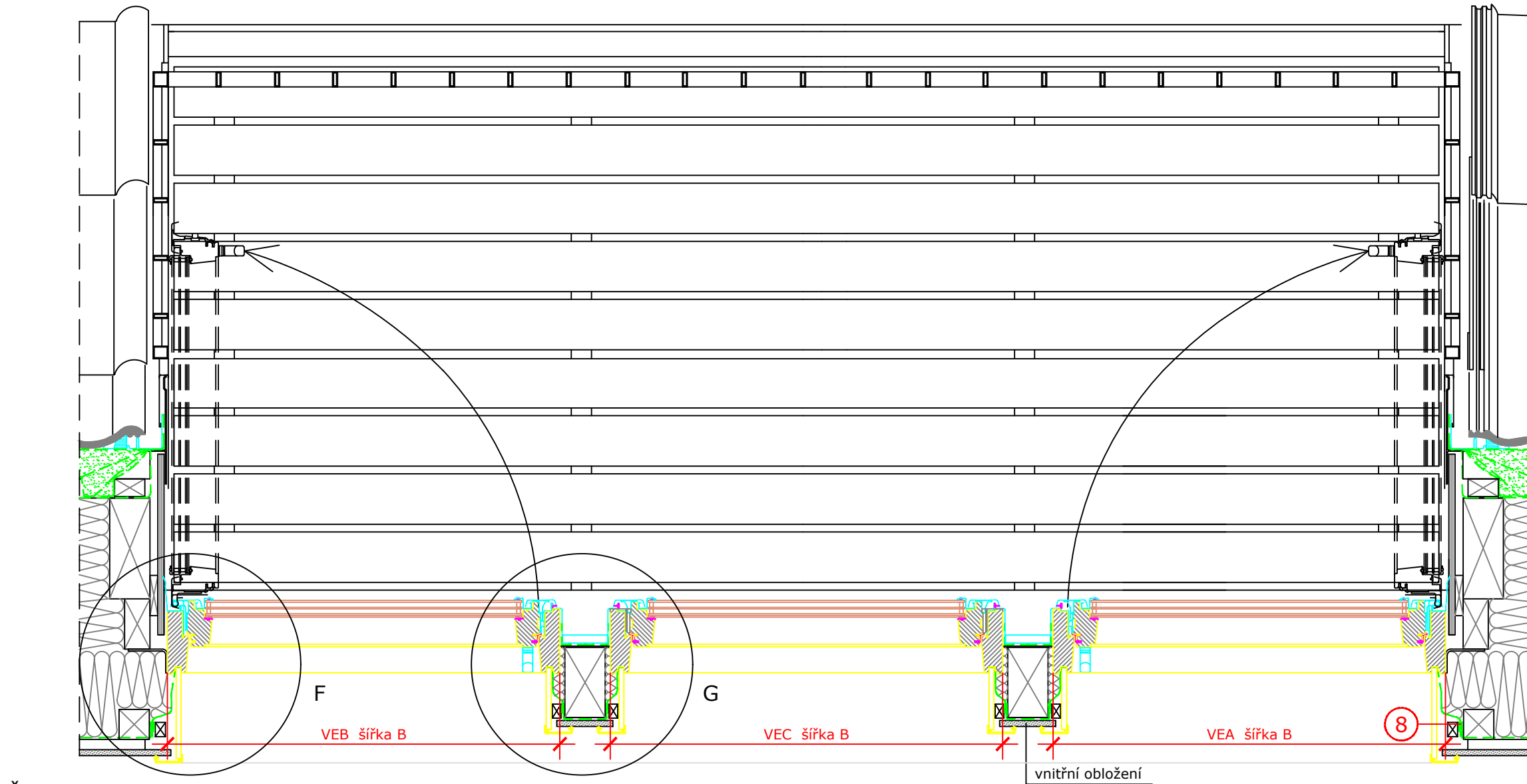
Řez spodním dílem střešní terasy GEL
