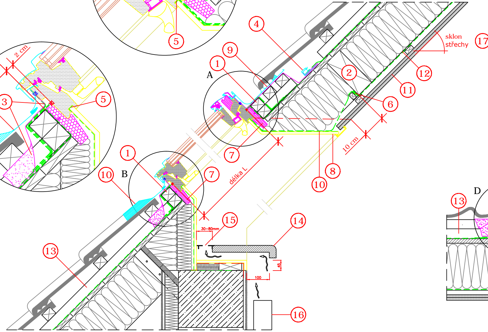
Řez A - A
