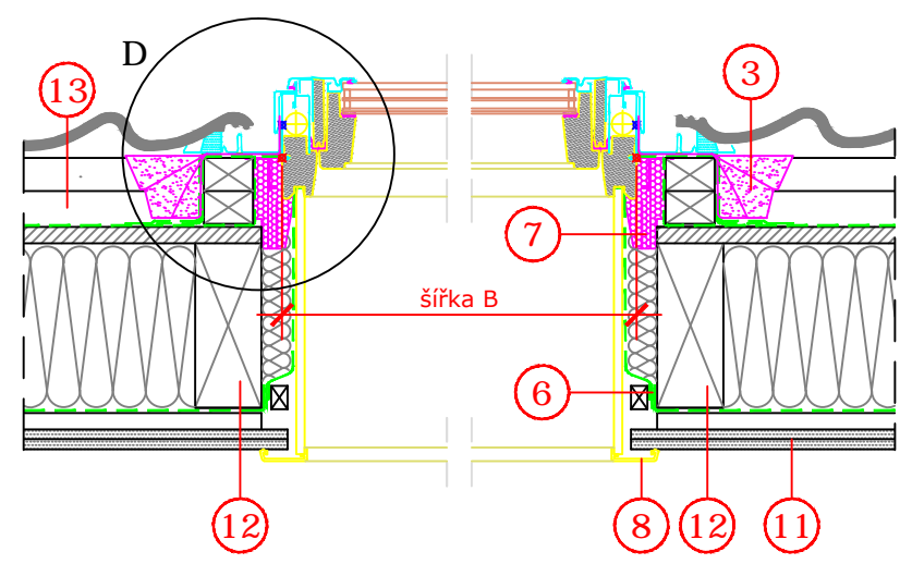
Řez B - B
