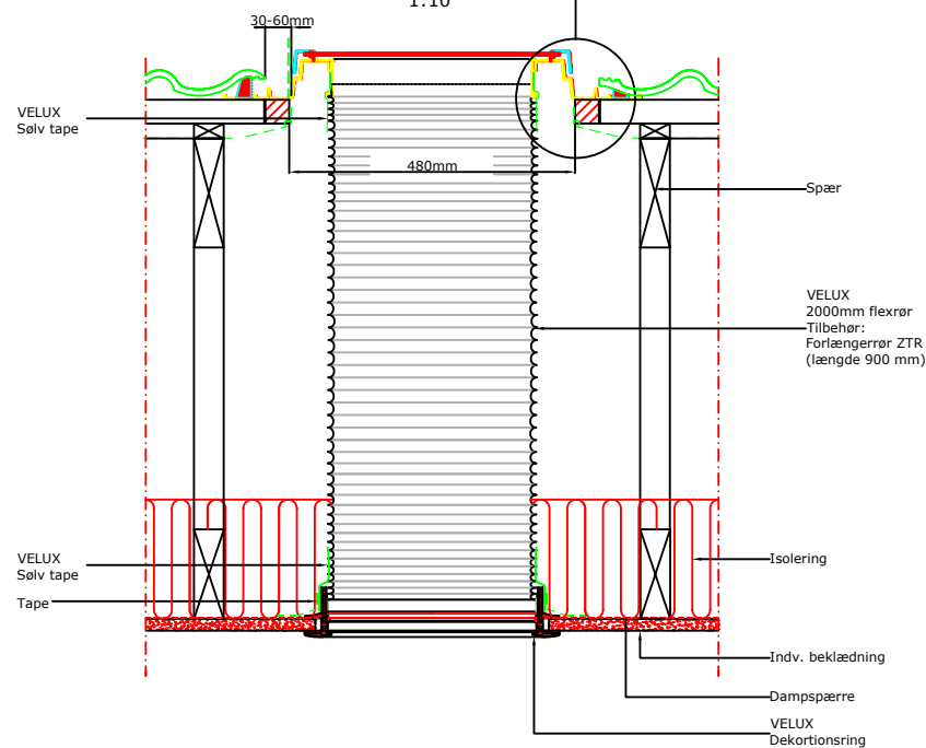
Snit B-B 1:10
