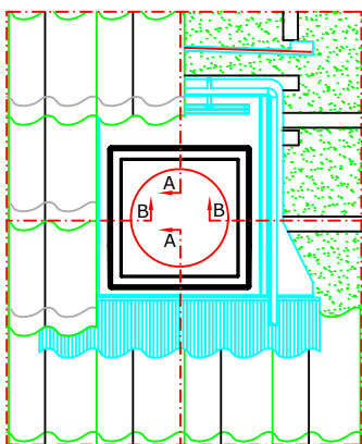
Opstalt vinkelret på tag 1:20
