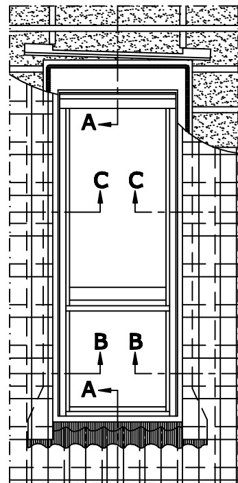
Eestvaade
