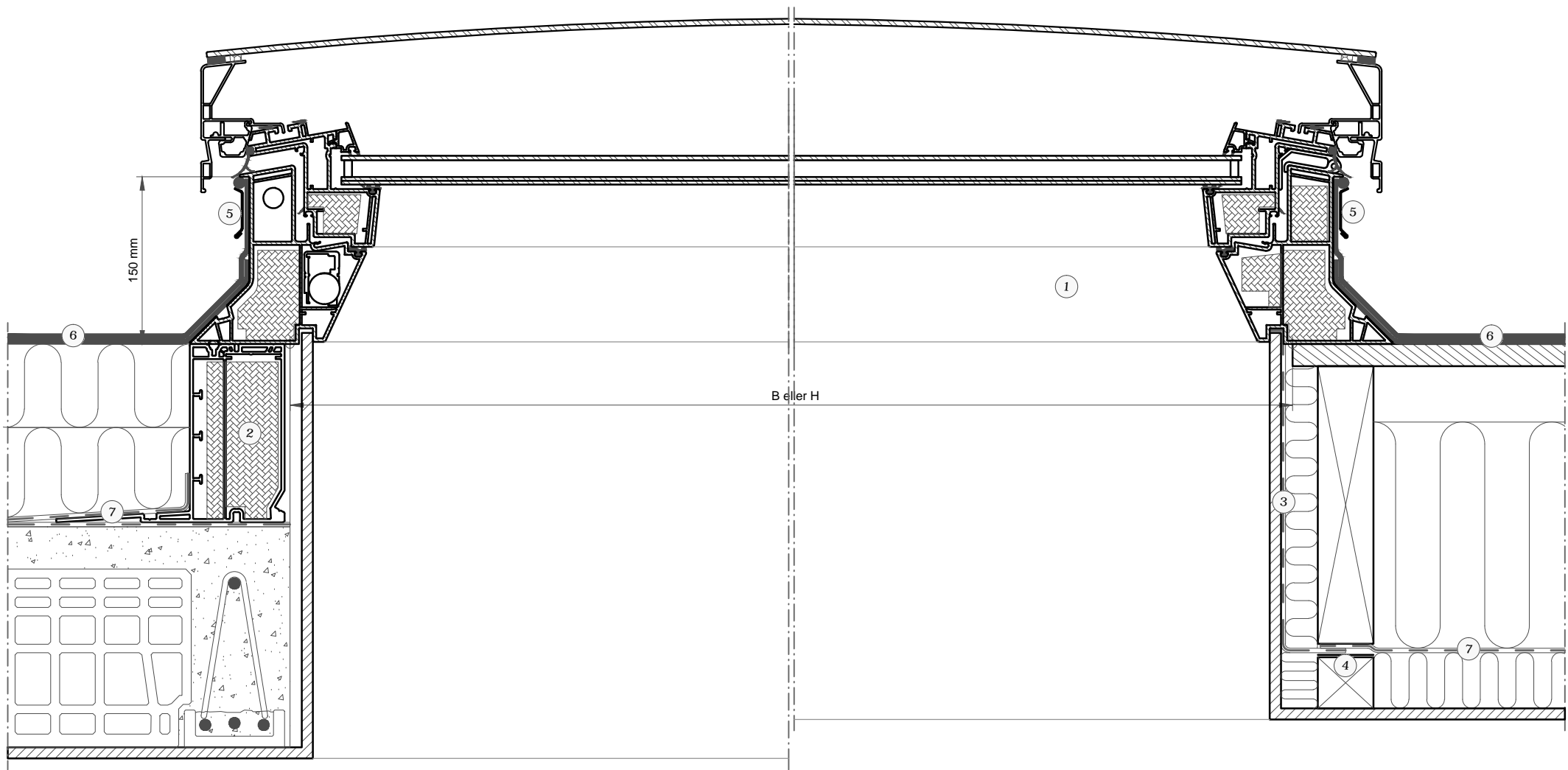
Snitt A-A 1:5
