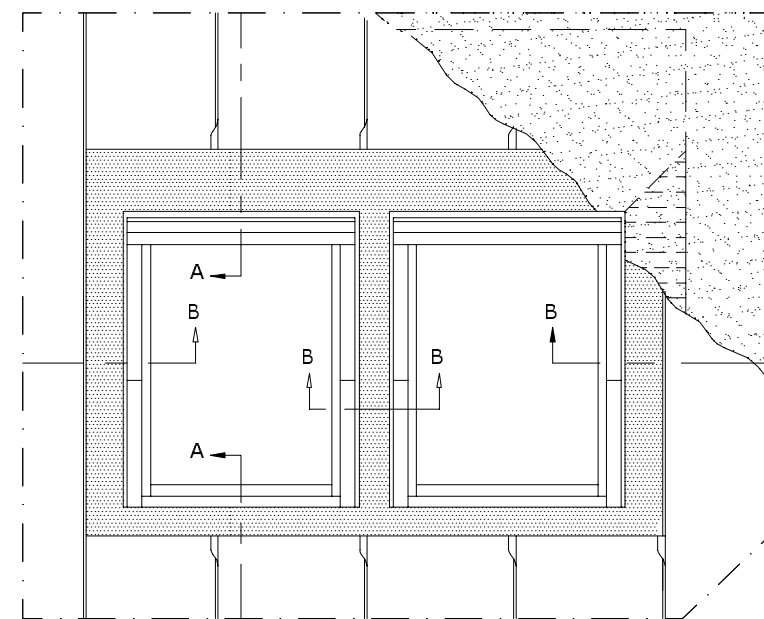
Section A-A 1:5
