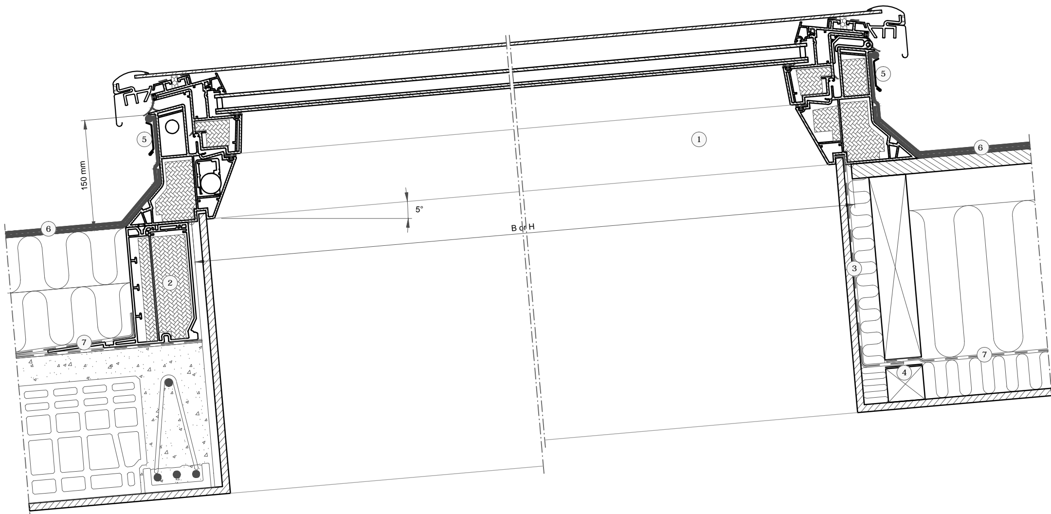
Snitt A-A 1:5
