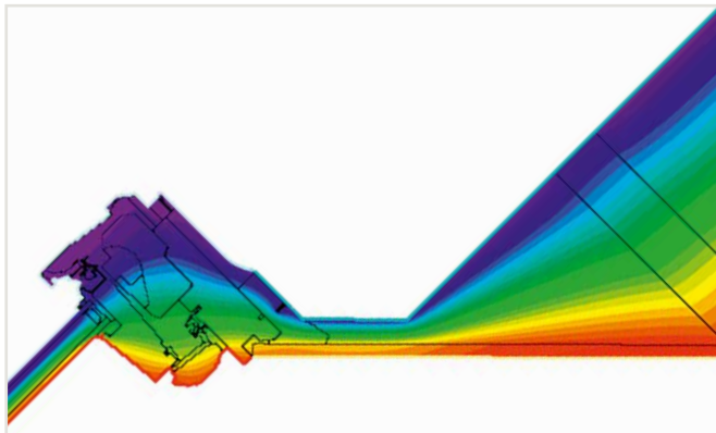
Montaż bez ramy izolacyjnej, wnela bez części prostopadłej do okna.
