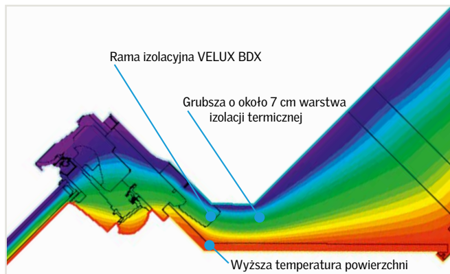
Montaż z ramą izolacyjną BDX i prawidłową, załamana wnelą okienną.
