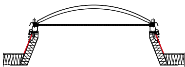
JET TOP-90 PLUS auf ISO-THERM Aufsetzkranz Ausstattungsoption Stellbleche (rote Linien)
