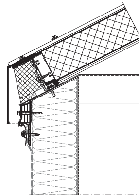
Traufanschluss (Längsseite) an einer Stahlzarge
