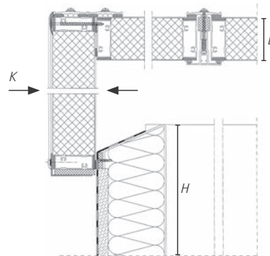
Giebelanschluss an einer Stahlzarge
