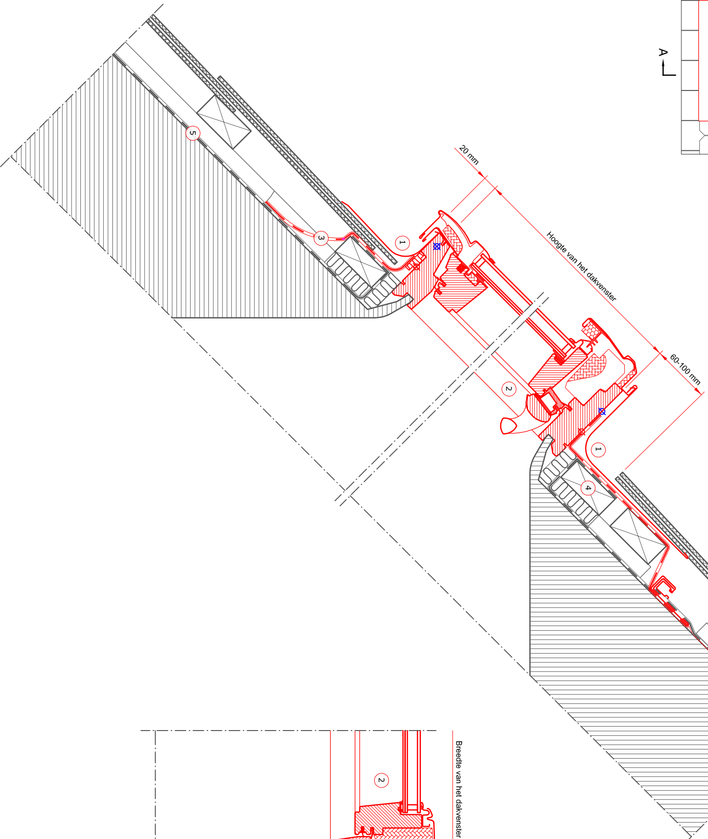
Doorsnede B-B 1:5
