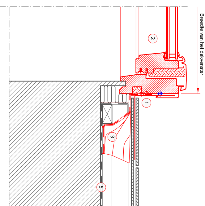
Doorsnede B-B 1:5
