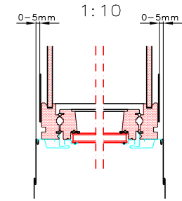
Coupe A-A
