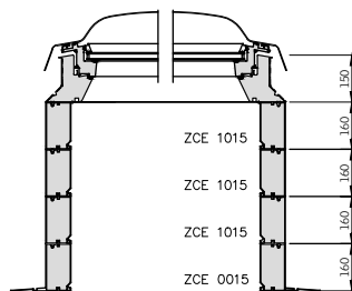
Flachdach-Fenster CVP/CFP mit Aufsetzkranz-Set ZCE S000, bestehend aus Aufsetzkranzen ZCE 0015 und ZCE 1015 + zusätzliche Aufsetzkranz-Adapter ZCE 1015. Es können bis zu drei Aufsetzkranz-Adapter ZCE 1015 gestapelt werden. Maximale Höhe 790 mm.
