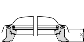
Flachdach-Fenster CVP/CFP
