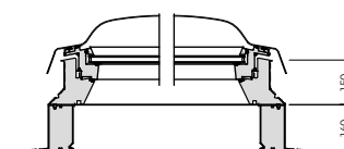
RWA Flachdach-Fenster CSP mit fix montiertem Aufsetzkranz
