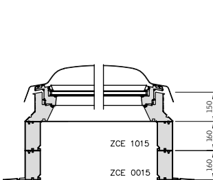
Flachdach-Fenster CVP/CFP mit Aufsetzkranzen ZCE 0015 und ZCE 1015 Set-Ausführung ZCE S000
