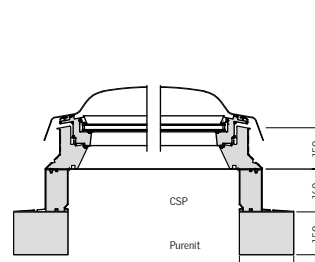
RWA Flachdach-Fenster CSP mit fix montiertem Aufsetzkranz mit zusätzlichem Purenit Aufsetzkranz
