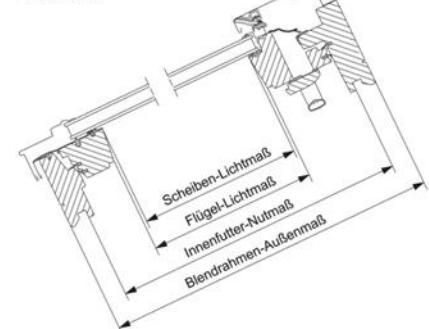
Längsschnitt
